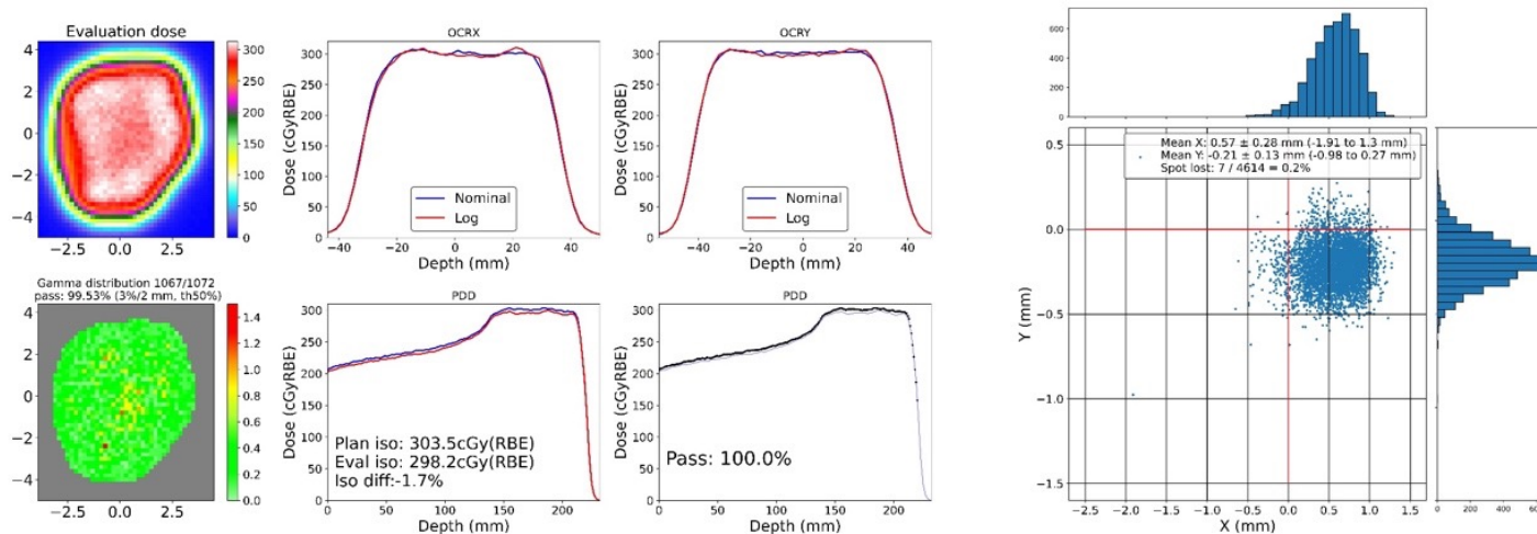
ログデータよりスポット位置を反映した線量分布(Log)と元のプラン(Nominal)の比較
